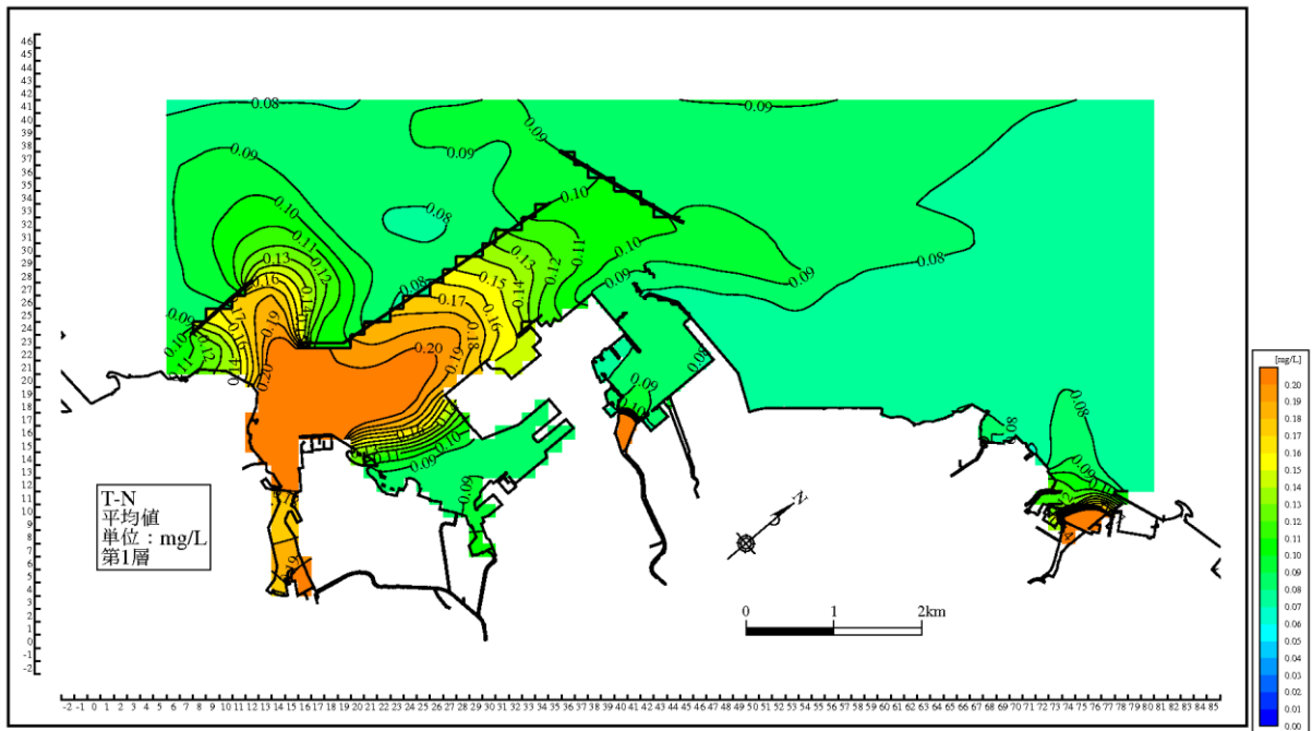
図 6.6.2.10(1) T-N 濃度分布の計算結果 (夏季, 平均潮, 日平均値, 第1層)
