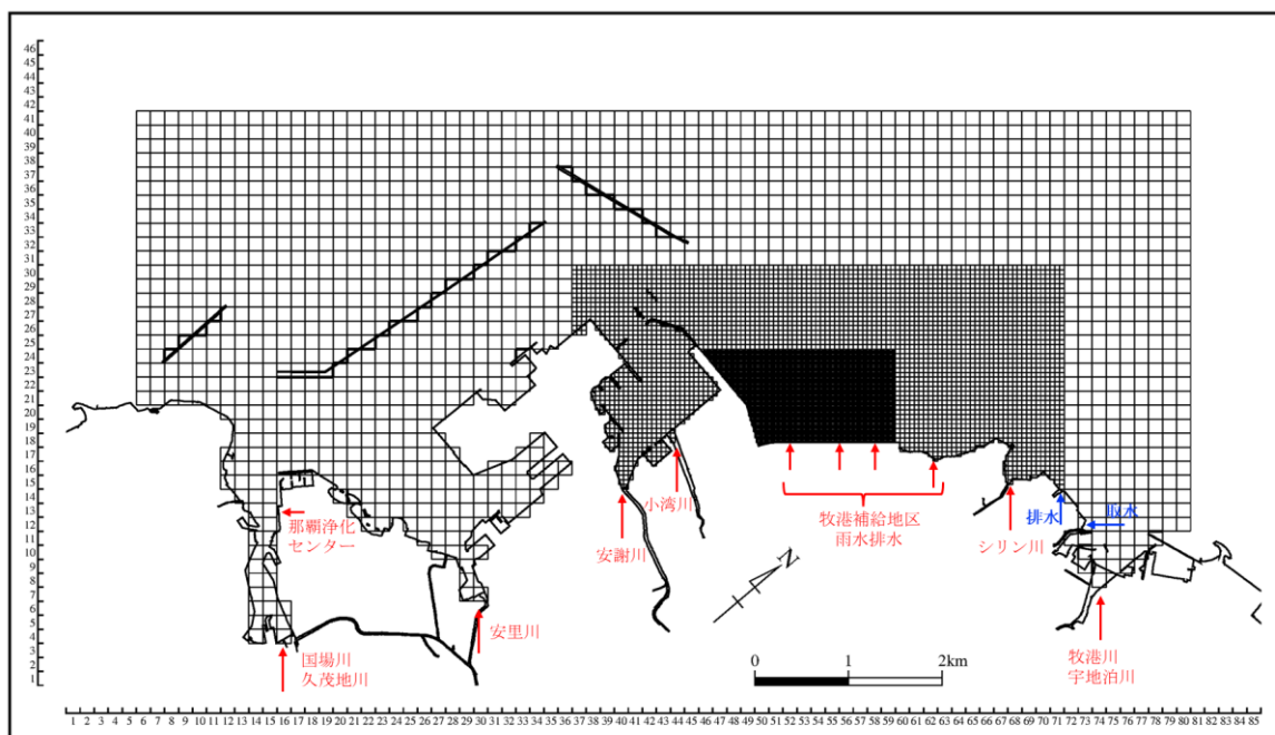
図 6.6.2.13(1) 降雨時の塩分の予測における計画なしの淡水流入位置 (大領域) (赤字：淡水流入、青字：発電所取排水)
