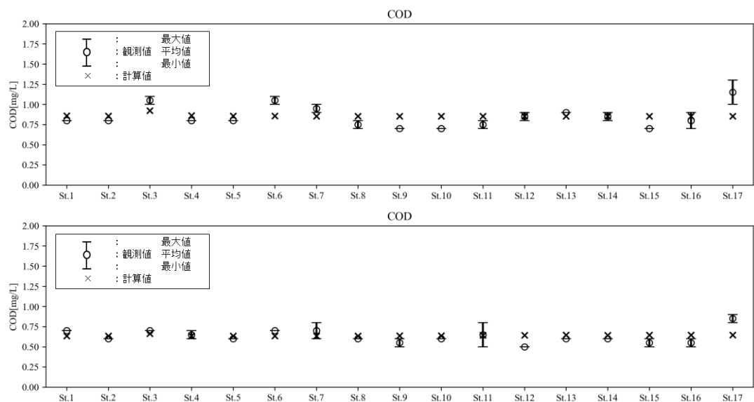
図 6.6.2.6 COD 濃度の観測値と計算値の比較（上：夏季、下：冬季）
