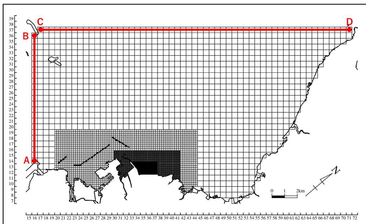
図 6.6.2.4 開境界の設定位置
