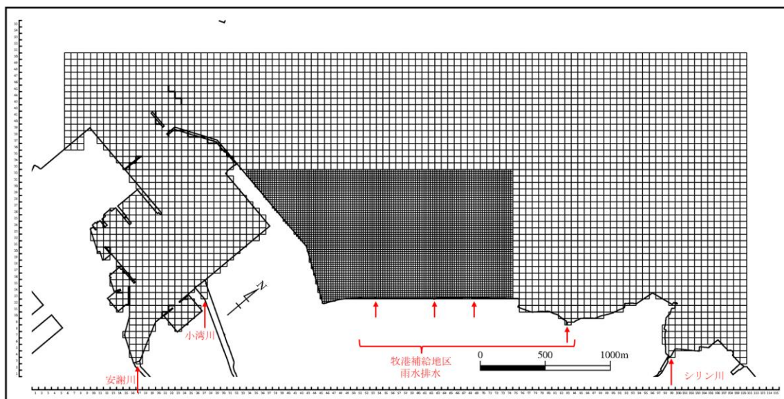
図 6.6.2.13(2) 降雨時の塩分の予測における計画なしの淡水流入位置 (中領域) (赤字：淡水流入、青字：発電所取排水)
