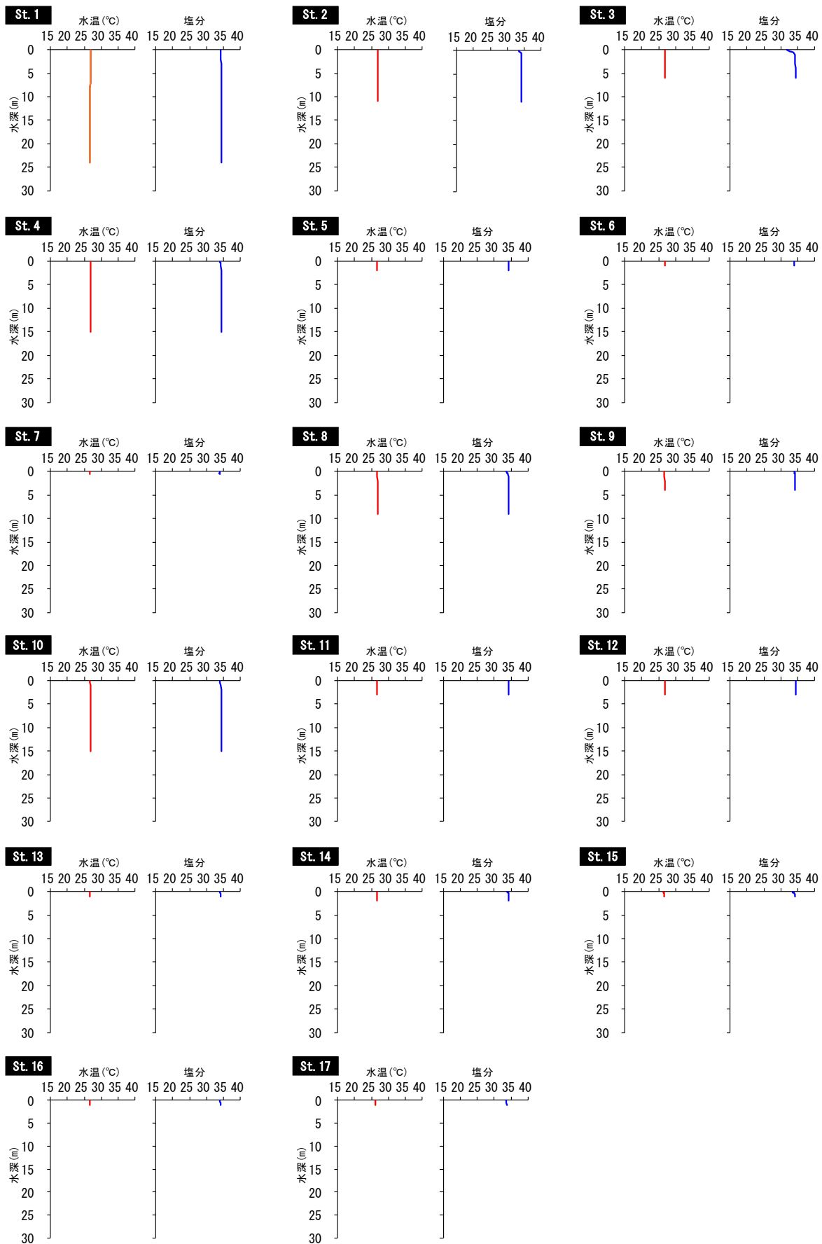
図 6. 6. 1. 4 (2) 水温・塩分の鉛直分布（平常時[下げ潮]、秋季、海域）
