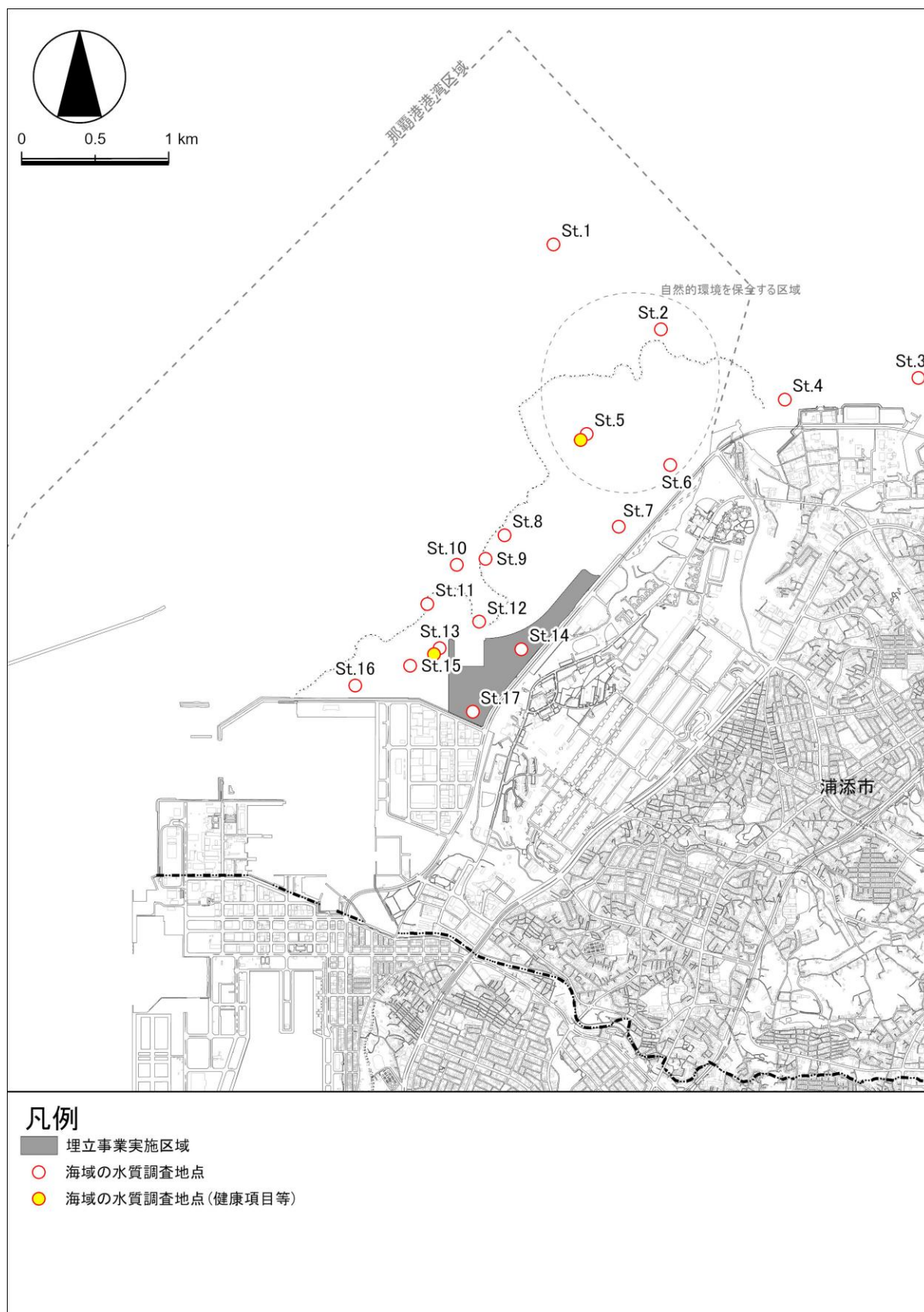
図 6.6.1.1 (1) 現地調査位置 (水質：海域)
