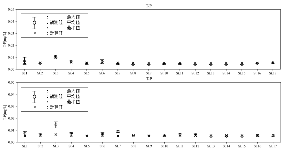
図 6.6.2.8 T-P 濃度の観測値と計算値の比較（上：夏季、下：冬季）
