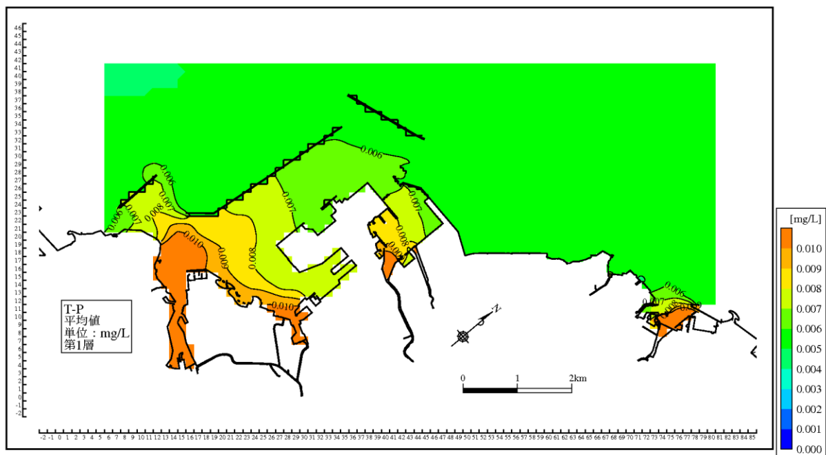
図 6.6.2.11(2) T-P 濃度分布の計算結果 (冬季, 平均潮, 日平均値, 第1層)
