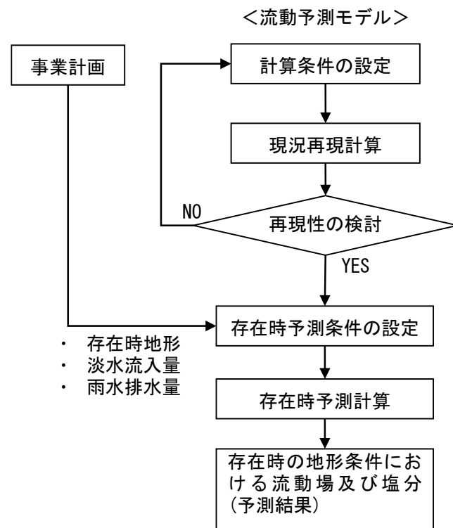
図 6.6.2.12 降雨時の塩分の予測手順
