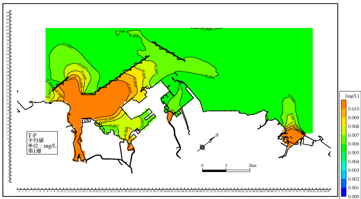
図 6.6.2.11(1) T-P 濃度分布の計算結果 (夏季, 平均潮, 日平均値, 第1層)
