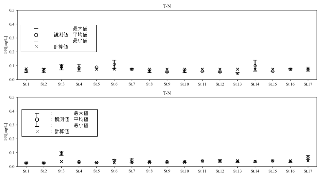
図 6.6.2.7 T-N 濃度の観測値と計算値の比較（上：夏季、下：冬季）
