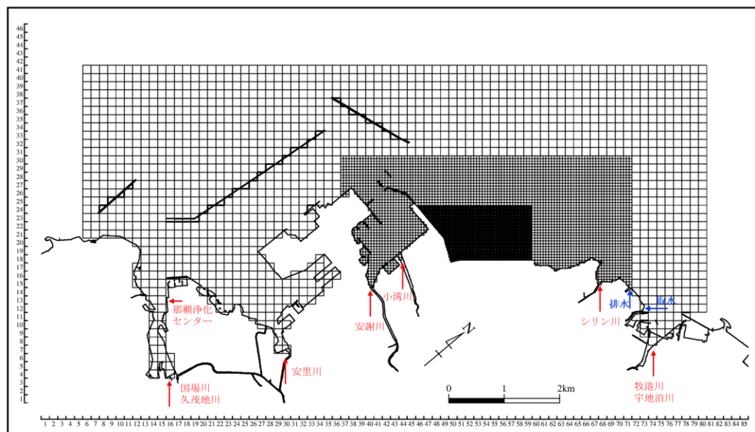
図 6.6.2.3 淡水流入の位置 (赤字：淡水流入、青字：発電所取排水)
