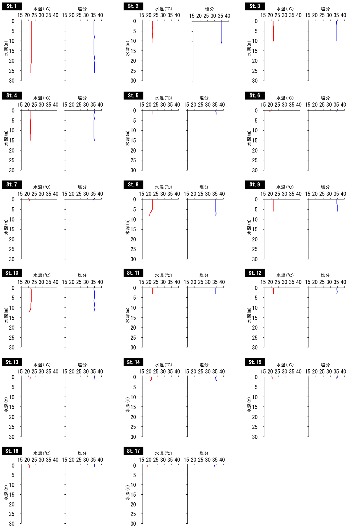
図 6.6.1.5(2) 水温・塩分の鉛直分布（平常時[下げ潮]、冬季、海域）
