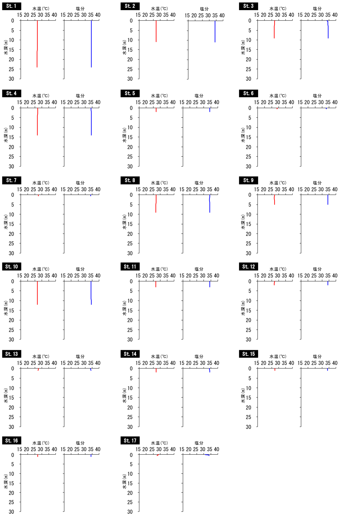
図 6. 6. 1. 4(1) 水温・塩分の鉛直分布（平常時[上げ潮]、秋季、海域）
