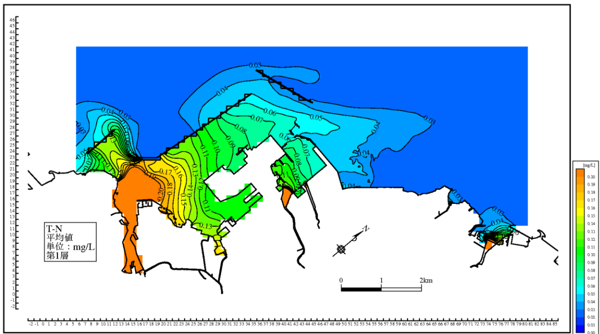
図 6.6.2.10(2) T-N 濃度分布の計算結果 (冬季, 平均潮, 日平均値, 第1層)
