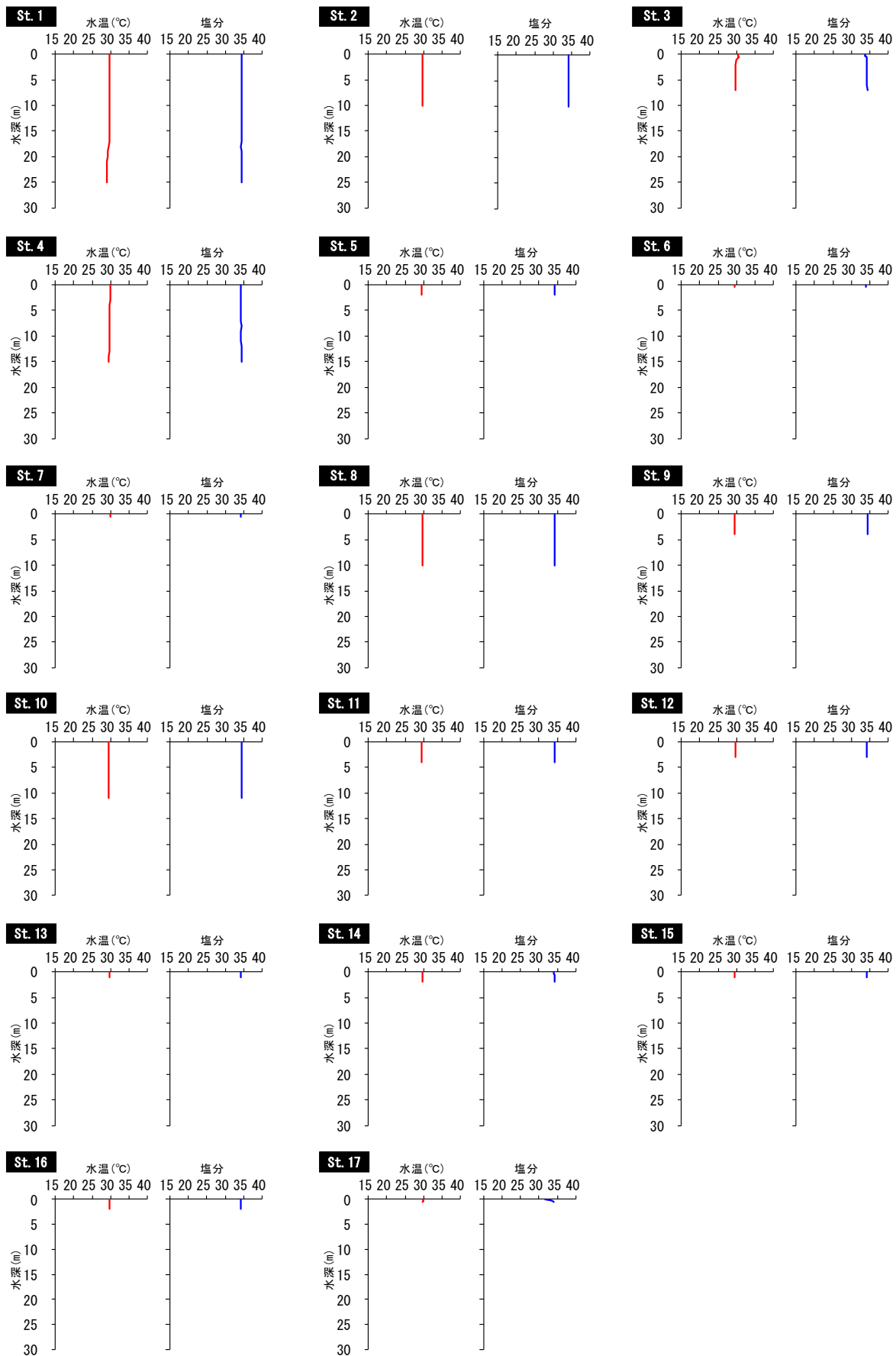
図 6. 6. 1. 3(1) 水温・塩分の鉛直分布（平常時[上げ潮]、夏季、海域）
