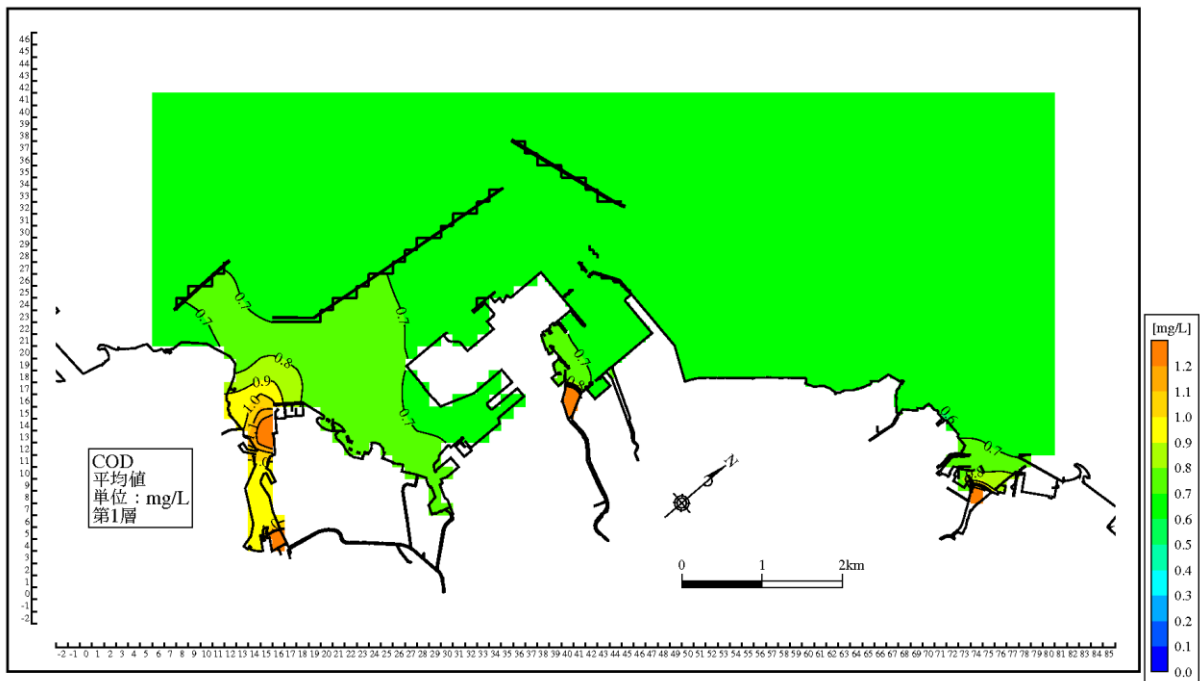
図 6.6.2.9(2) COD 濃度分布の計算結果 (冬季, 平均潮, 日平均値, 第 1 層)
