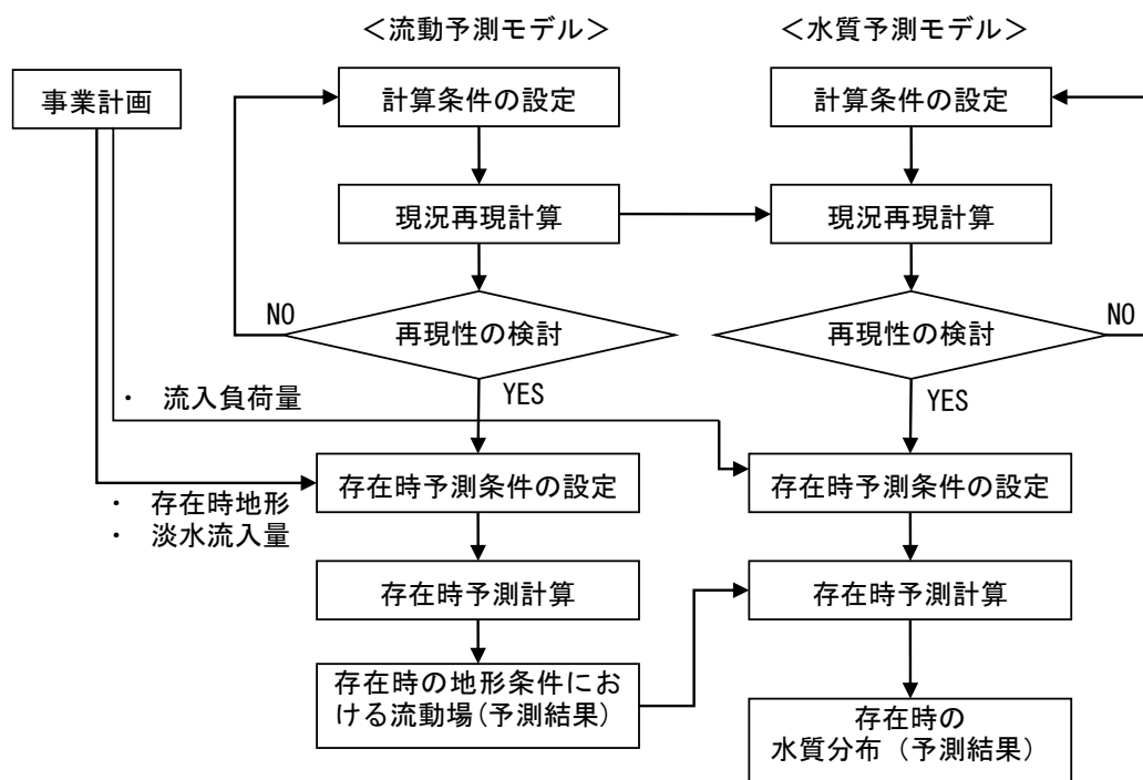
図 6.6.2.2 COD、T-N、T-P の予測手順
