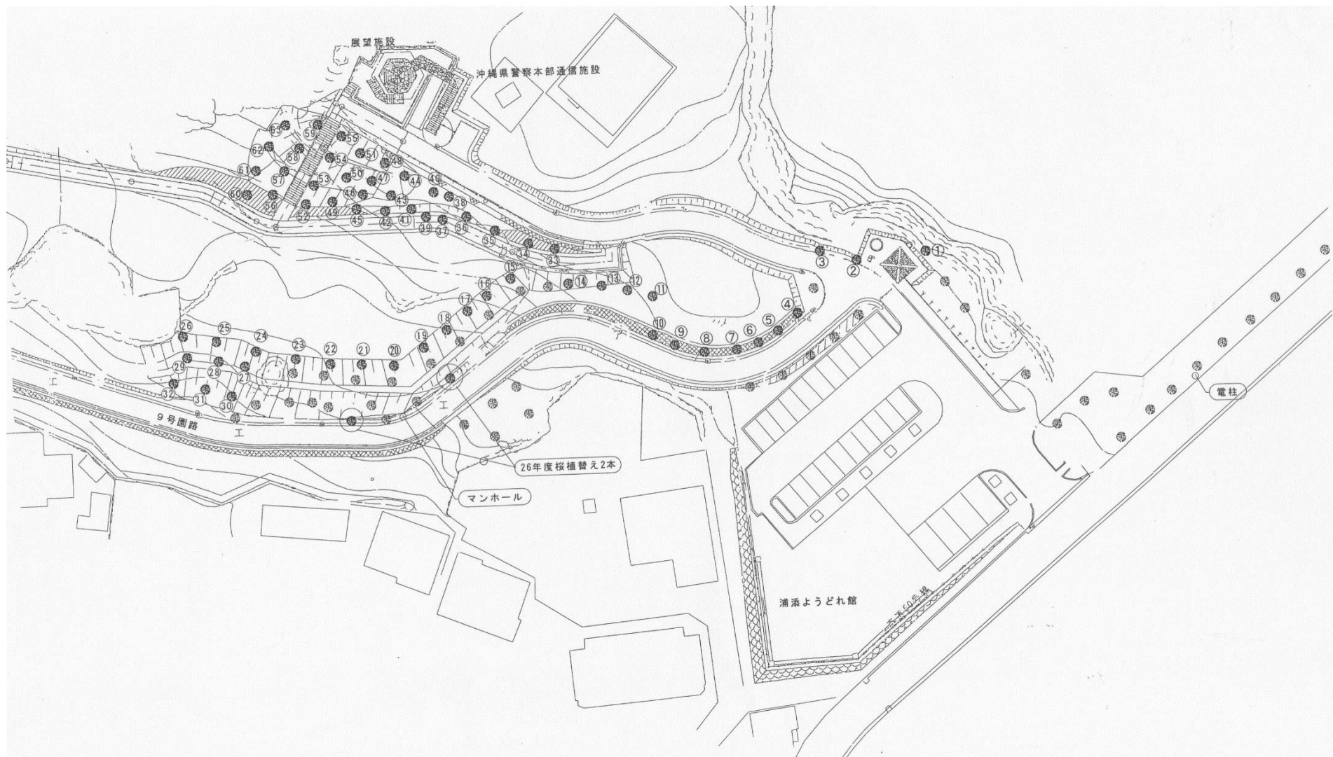
平成26度桜植栽計画図
