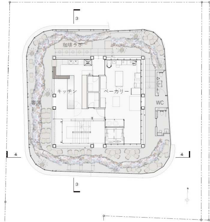
2L 階平面図
