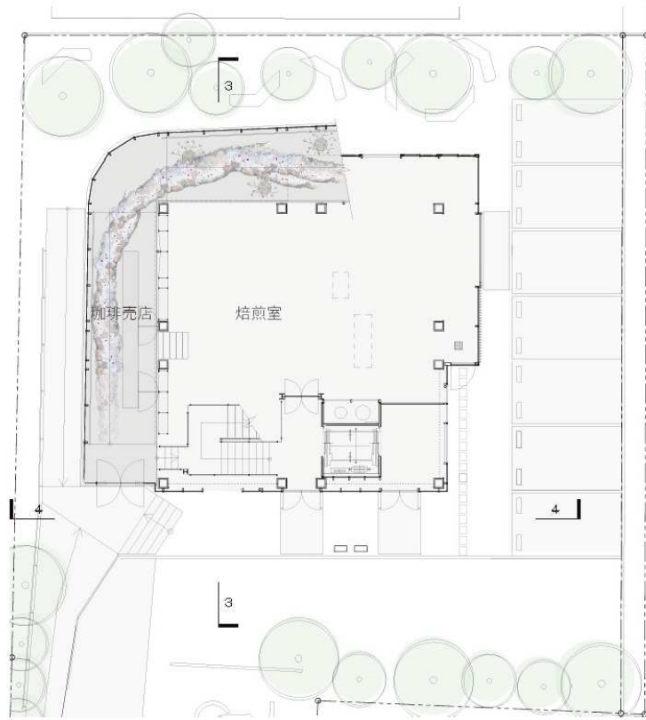
一階平面図
