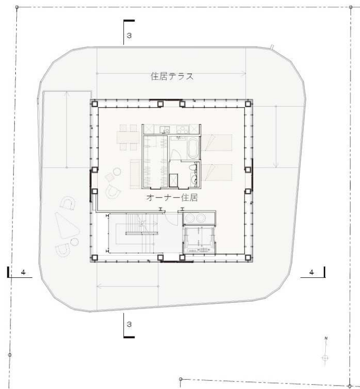
3 階平面図
