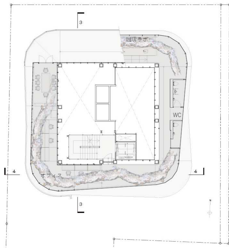
20 階平面図
