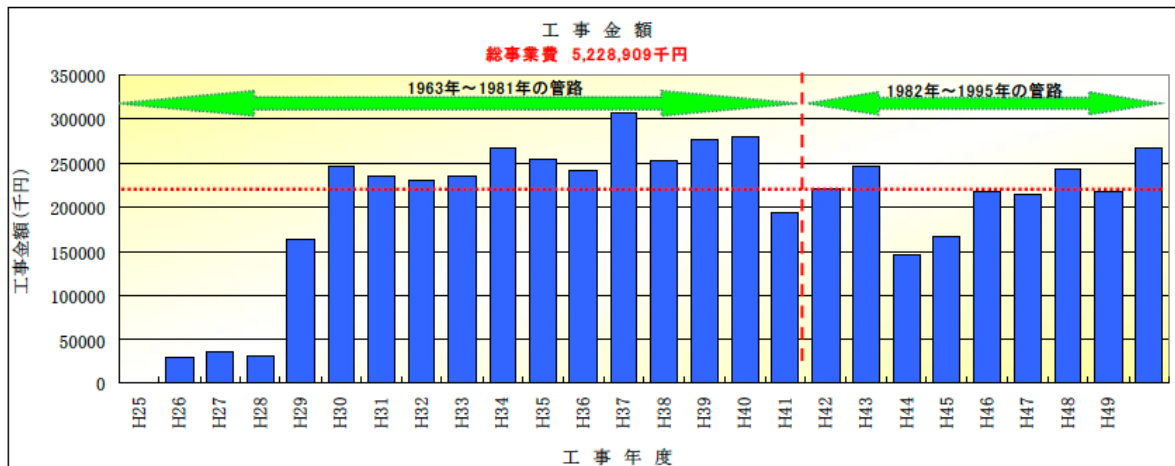
図10 上水道の将来コストと長寿命化
