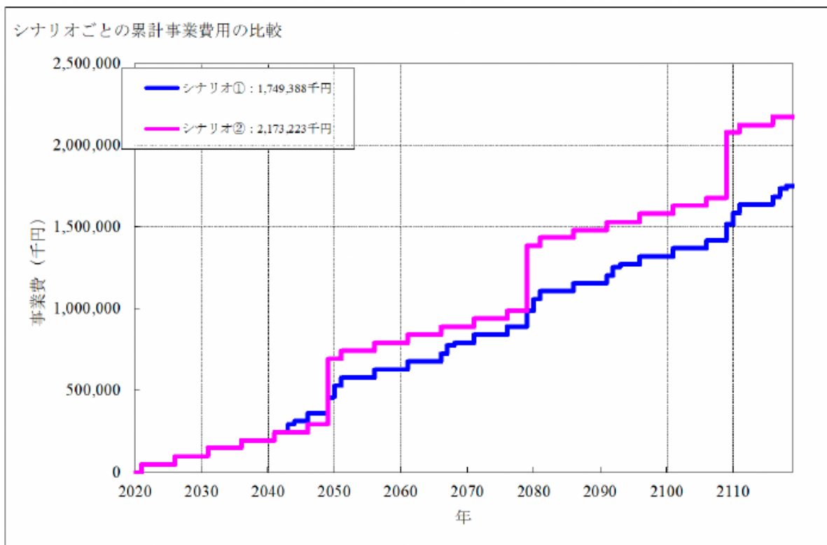
図8 モノレールの予防保全と長寿命化
