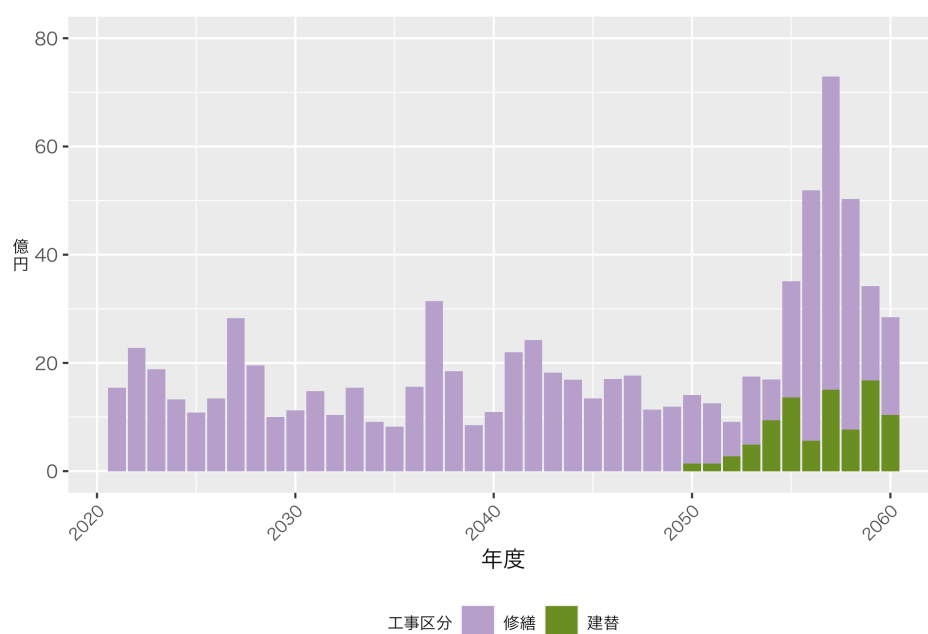
図6 建物将来コスト 長寿命化
