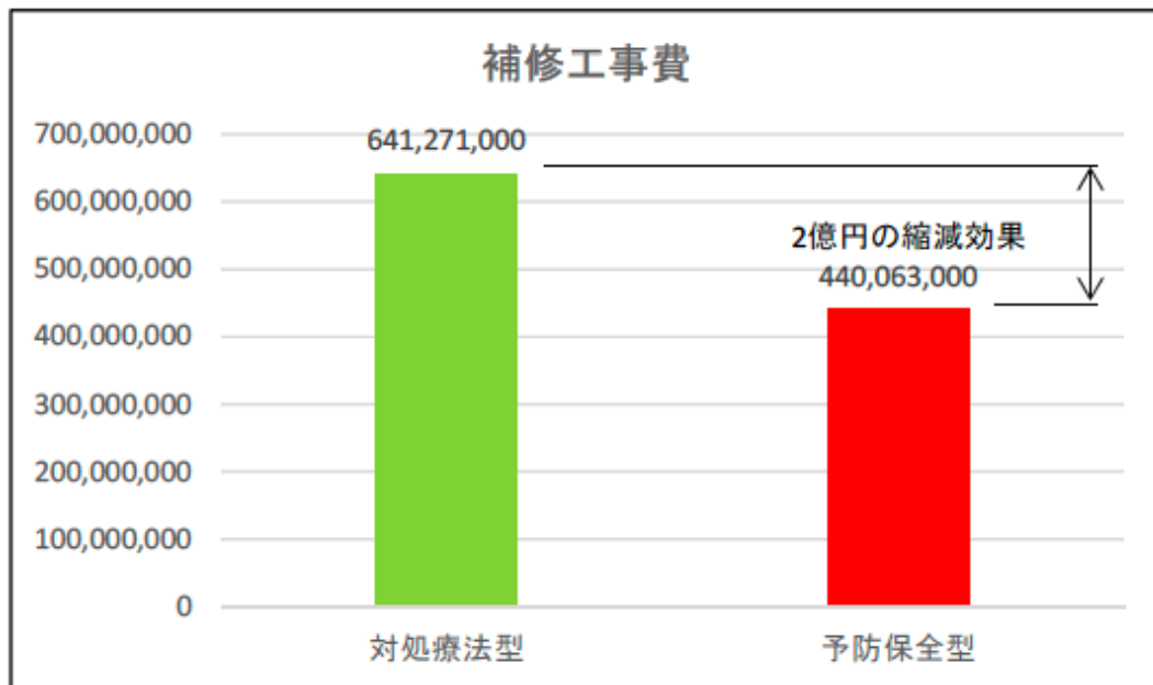
図7 道路の補修工事と長寿命化
