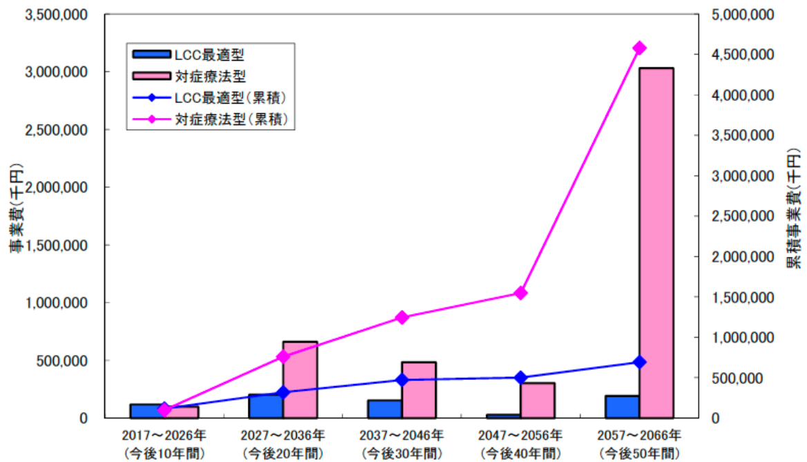
図9 橋りょうの将来コストと長寿命化
