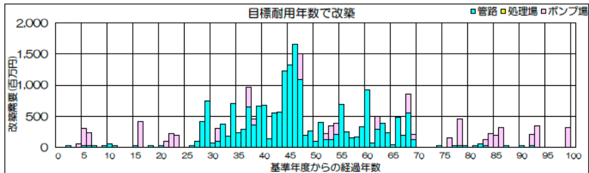
図11 下水道の LCC と長寿命化
